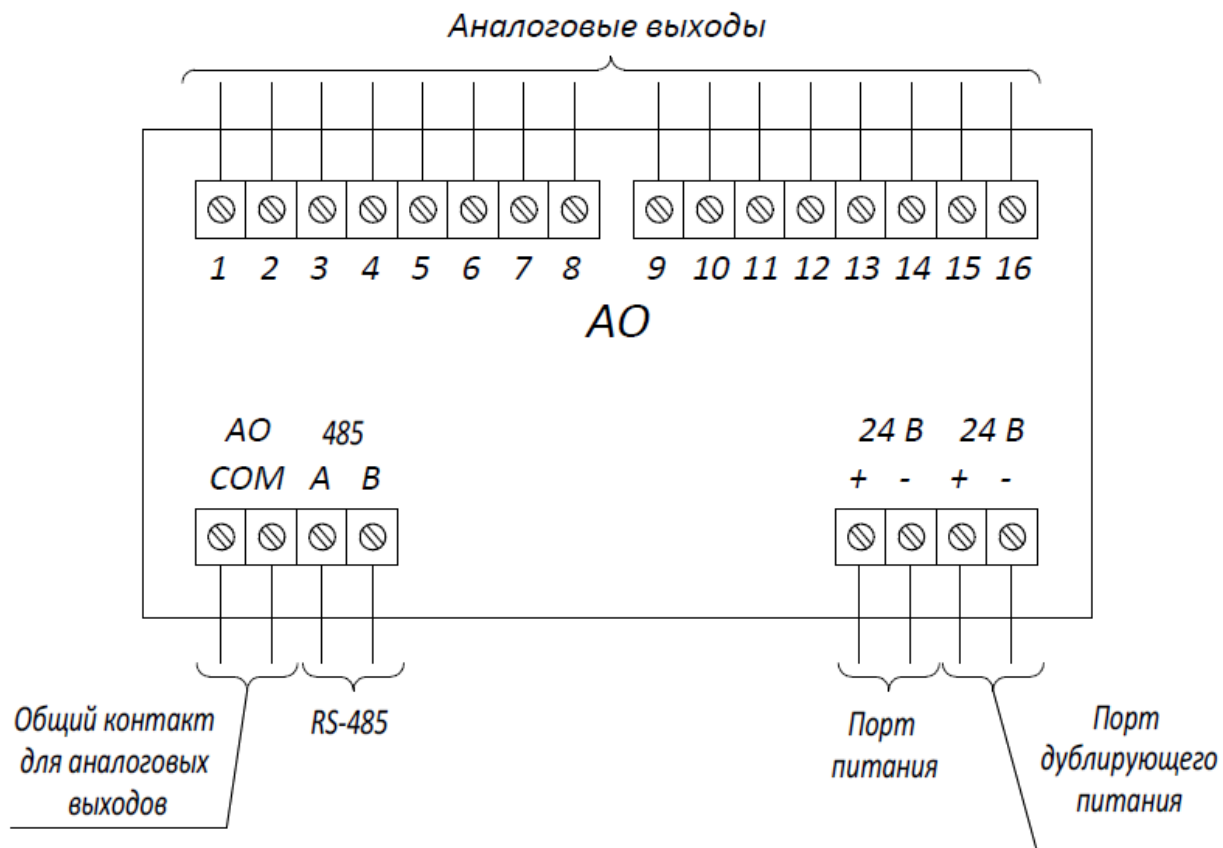
Рисунок 5.1 – Назначение контактов клеммников.
