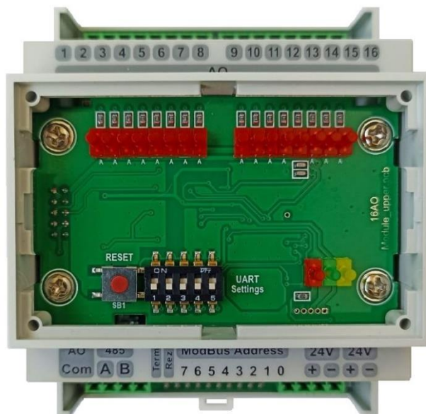
Рисунок 5.3 – Прибор со снятой крышкой лицевой панели.
