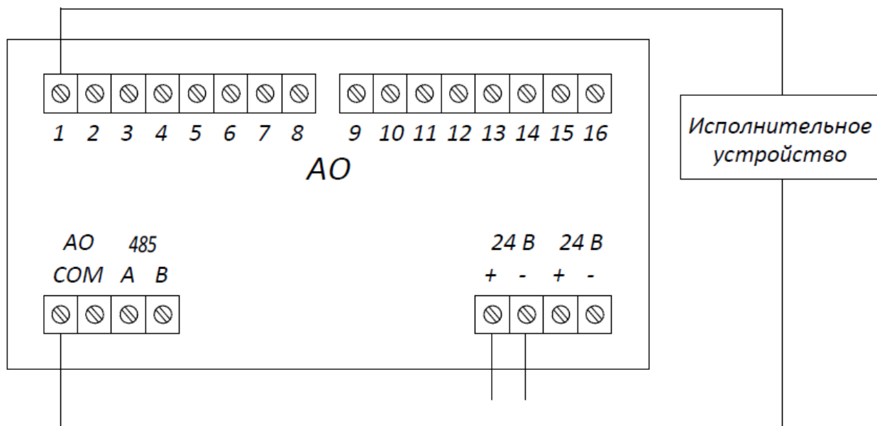
Рисунок 5.2 – Подключение к аналоговым выходам.
