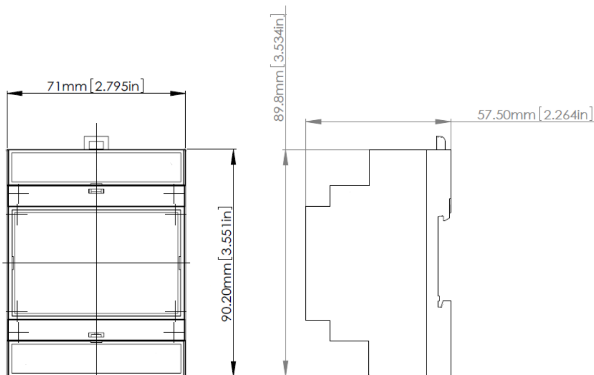
Рисунок 4.1 – Габаритные размеры.
